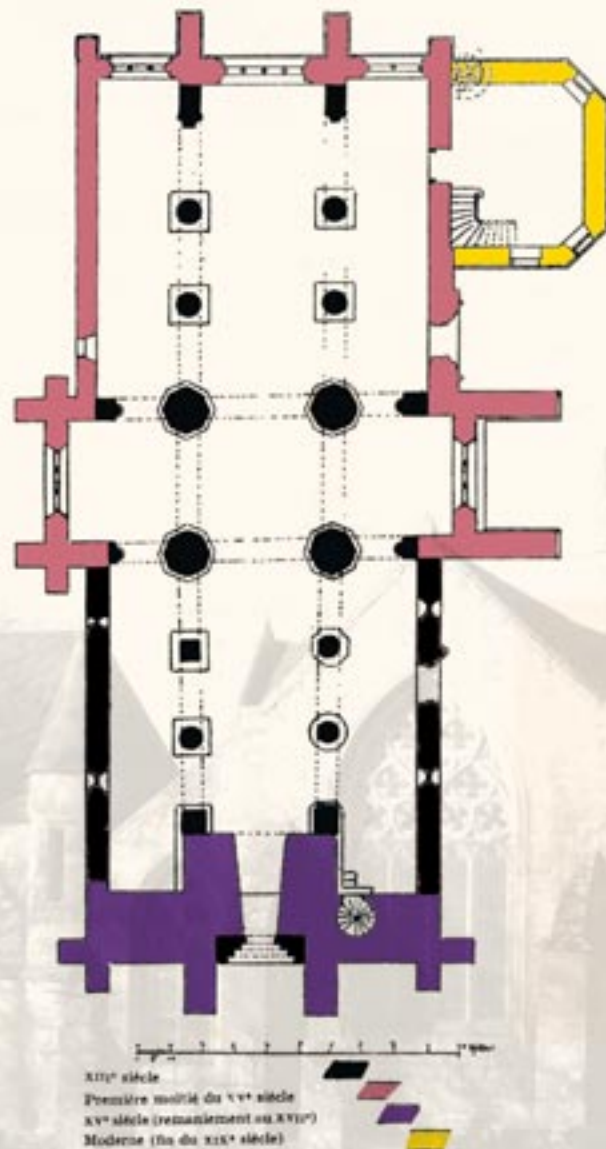
Plan de la Chapelle de Kerinec (Ch Chaussepied, architecte)
